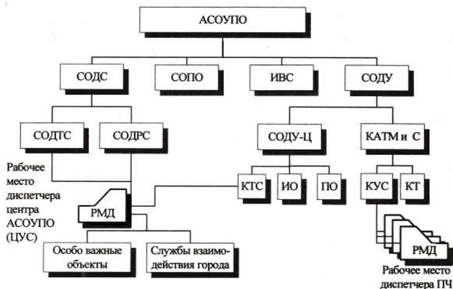
Рисунок 1. Структурная схема АСОУПО
